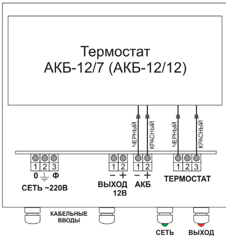
Рисунок 2. Стандартный вариант подключения термостата АКБ к источнику (без отключения термостатирования в режиме «Резерв»)
