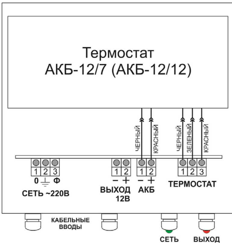
Рисунок 3. Экономичный вариант подключения термостата АКБ к источнику (с отключением термостатирования в режиме «Резерв»)
