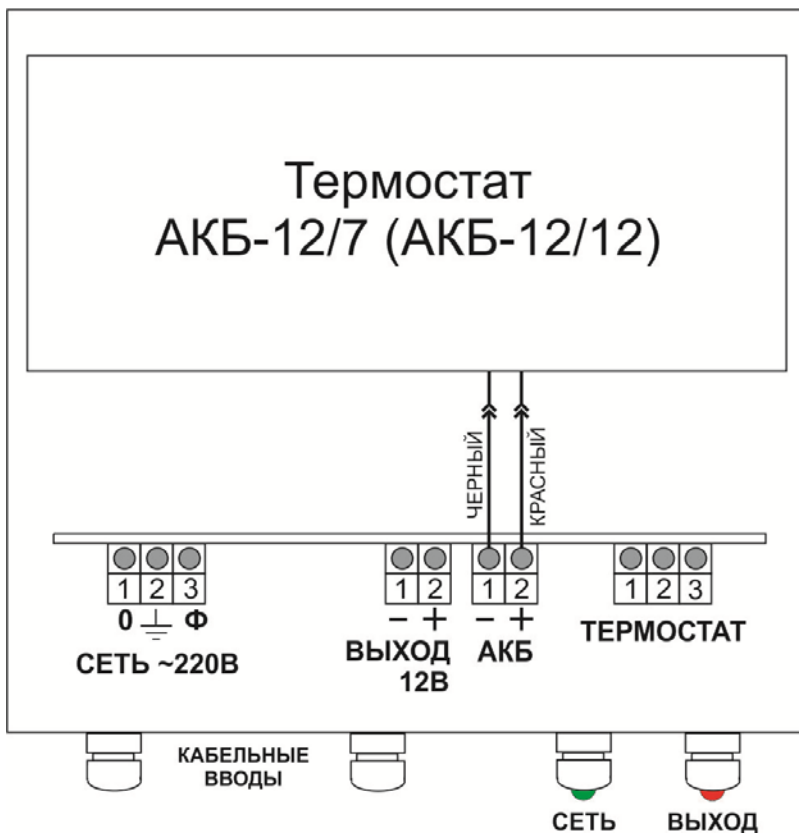
Рисунок 1. Вид источника с открытой крышкой (схема подключения)
