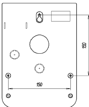
Расположение отверстий для крепления на основании «АС-Р2»
