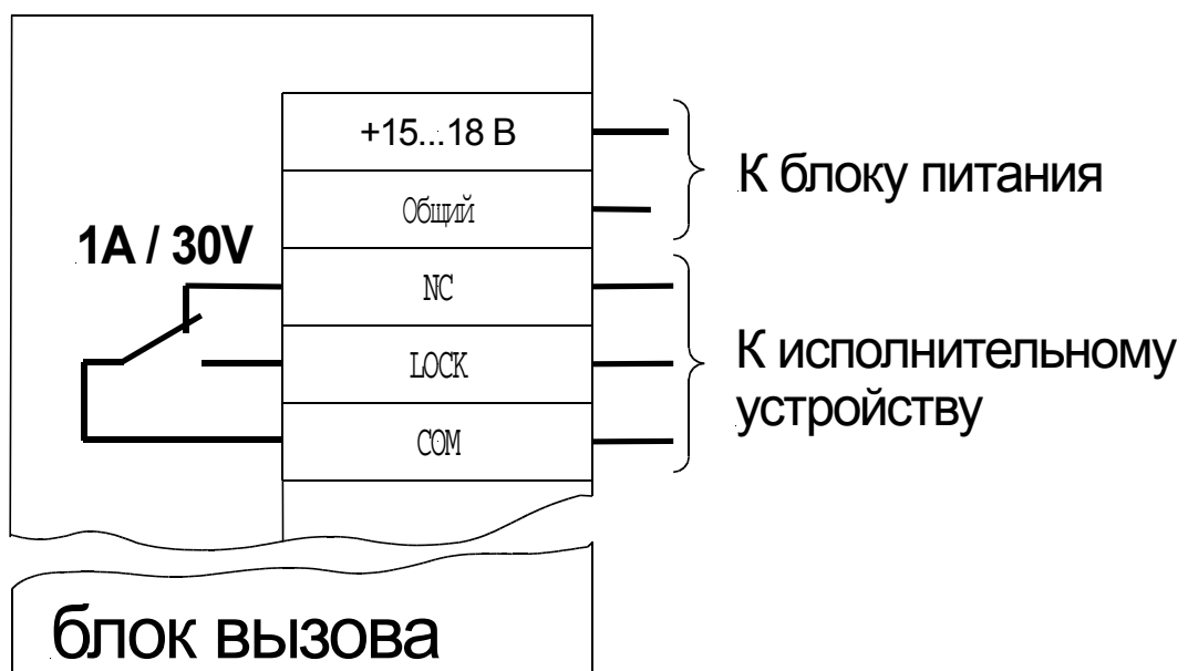
Рис. 4. Подключение замка с платой управления или исполнительного устройства к блокам вызова моделей М10.1-ТМ4 R
