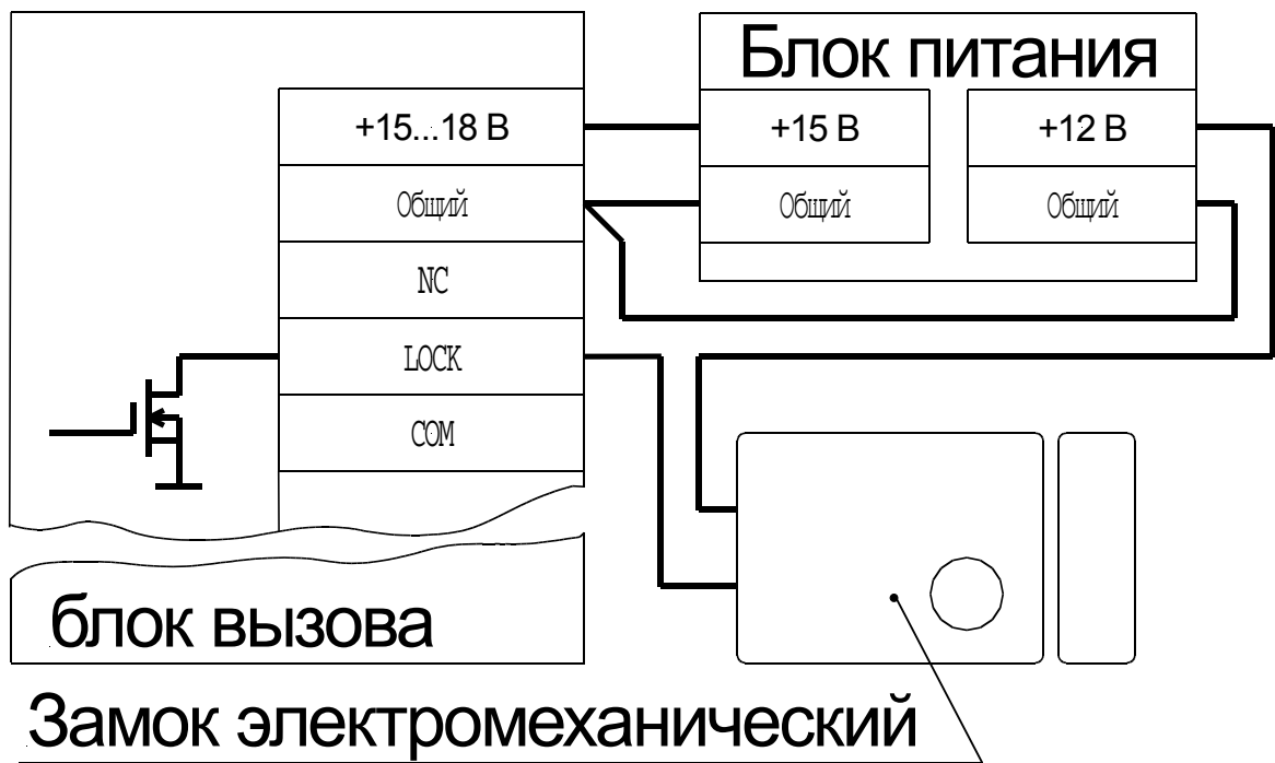
Рис. 3. Подключение электромеханического замка к блокам вызова моделей М10.1-ТМ4 М.
