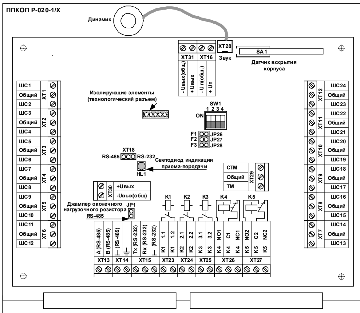
Рис. 16 Прибор исполнения Р-020-1/Х-Х (без БП)
