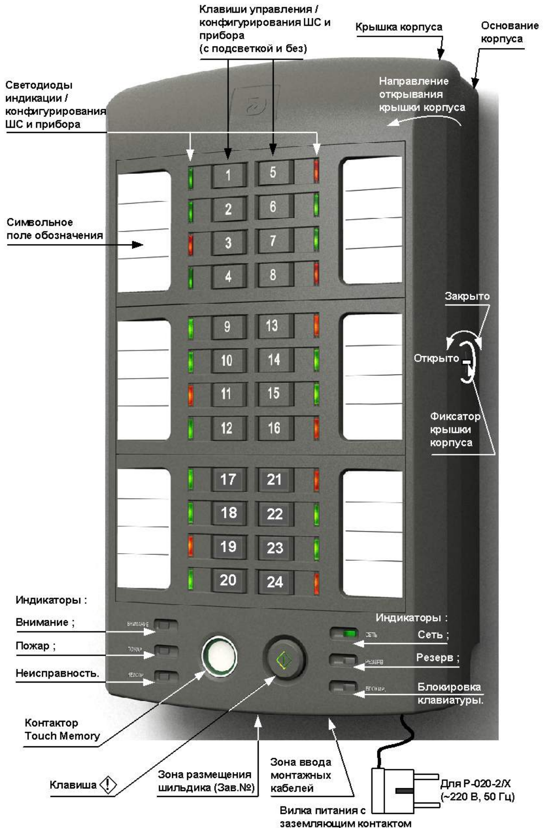
Рис. 1 Внешний вид прибора
