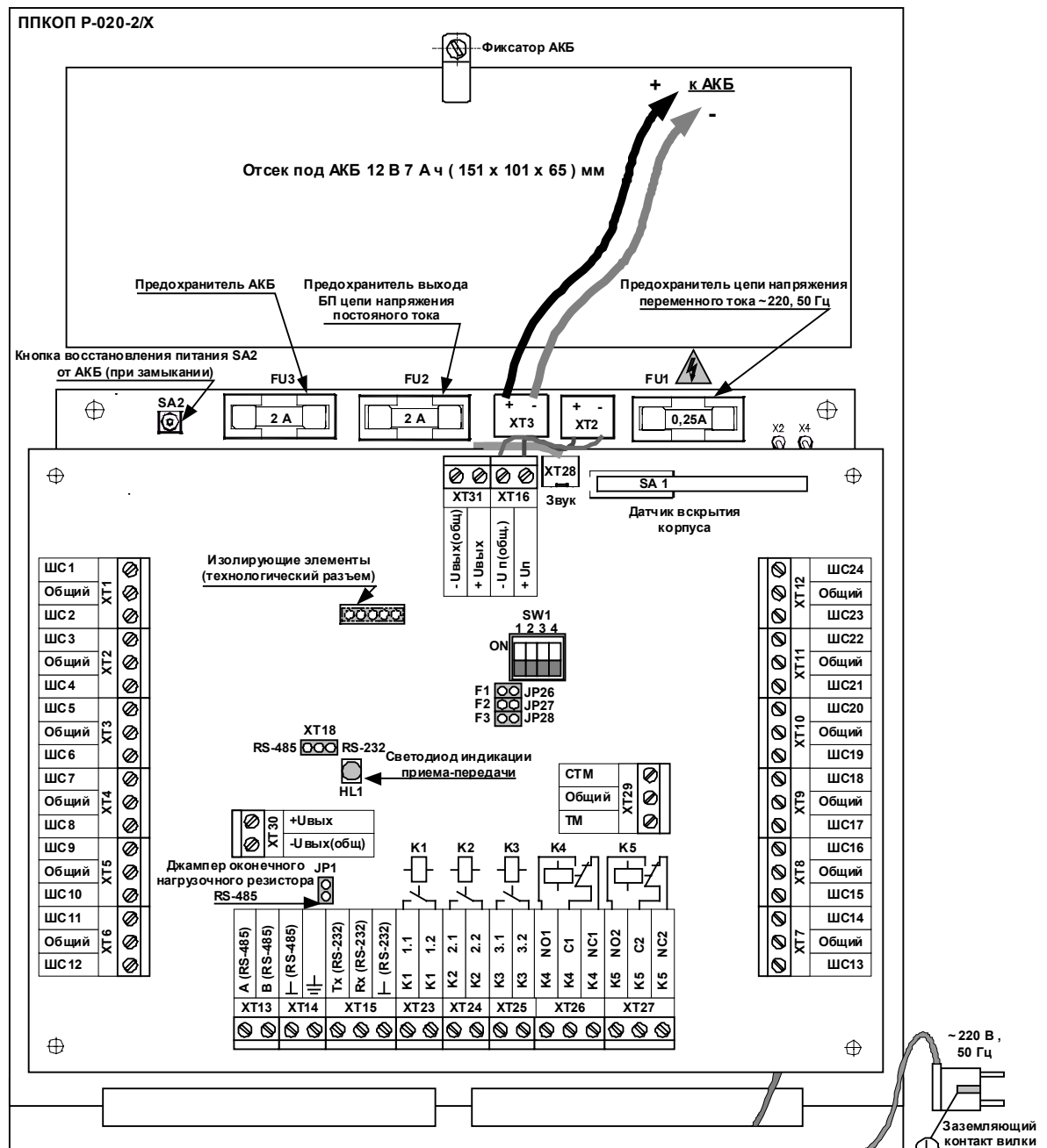
Рис. 17 Прибор исполнения Р-020-2/Х-Х (с БП)
