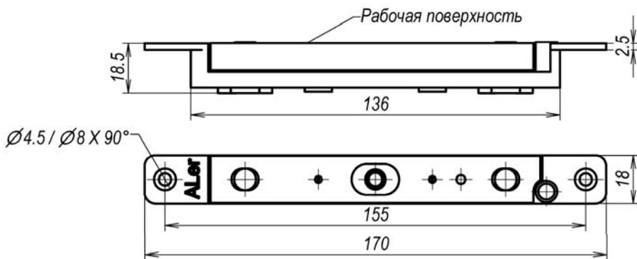
Рис.4 Якорная часть
