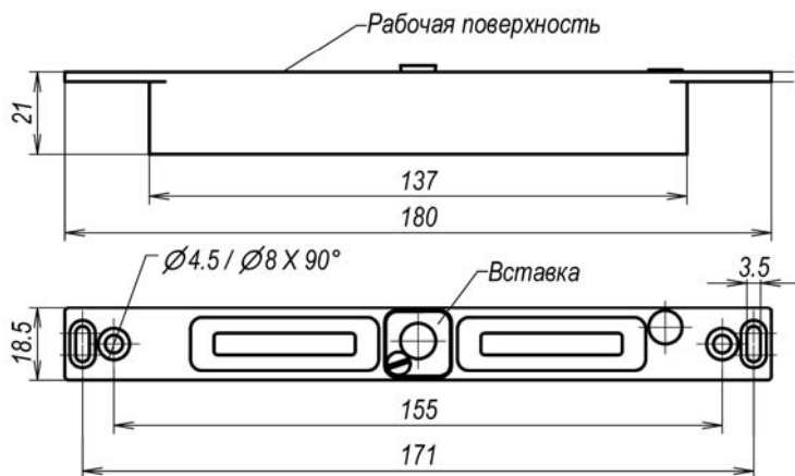
Рис.5 Корпусная часть
