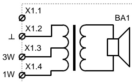
Схема электрическая оповещателя речевого «Соната-Т» исп.2- рис.1
