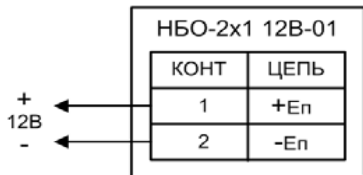
Рис.1 Схема подключения.
