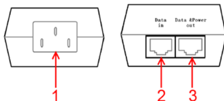
Рис. 2 Элементы Midspan – 1/36(60)
