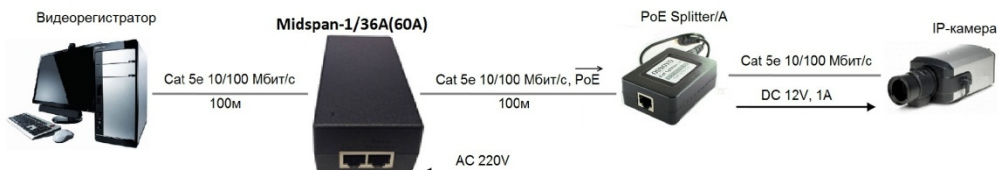
Рис. 3 Схема подключения PoE-инжекторов Midspan – 1/36A(60A)
