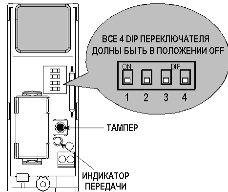
Рисунок 6. Открытие корпуса
