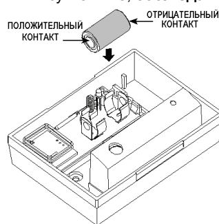
Рисунок 7. Установка батареи
