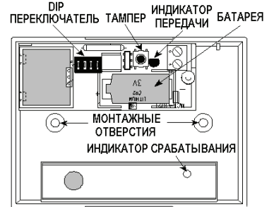
Рисунок 2. Вид изнутри
