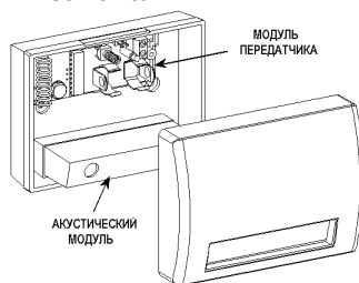
Рисунок 2. Расположение модулей
