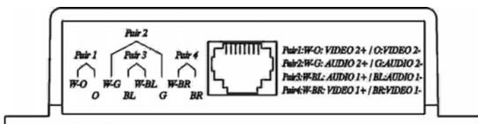
Задняя панель
