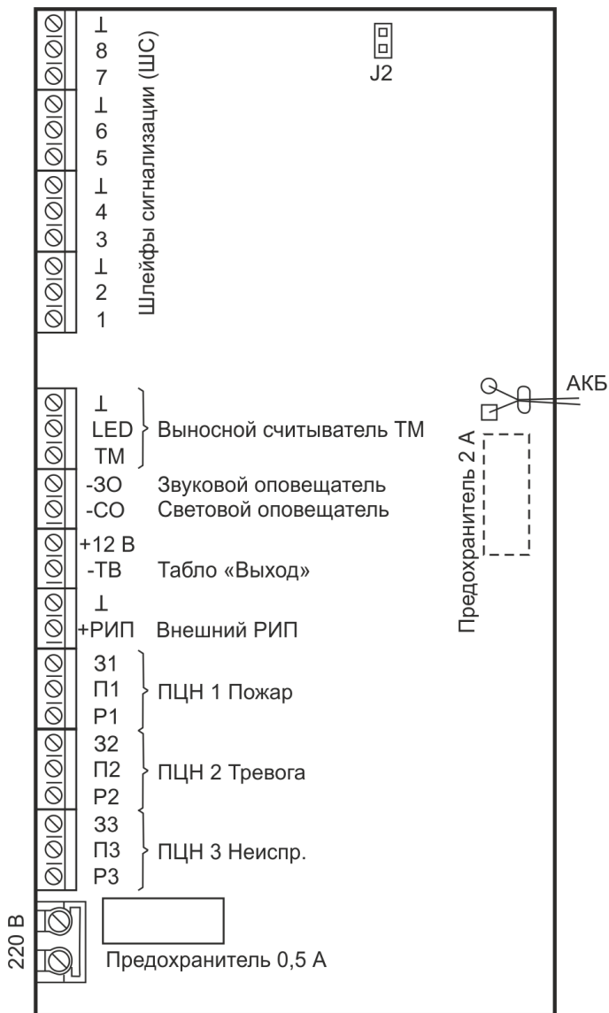
Рис.10. Вид на клеммы и разъемы для внешних подключений ВС-ПК2(4,8)(Т) версия 2.0.
