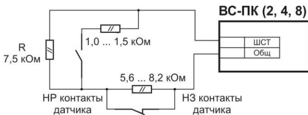
Рис.7. Схема включения технологических датчиков в ШСТ. НР – нормально разомкнутые контакты датчика НЗ – нормально замкнутые контакты датчика
