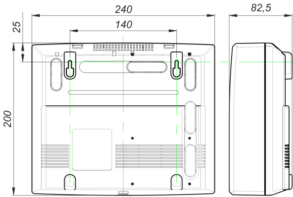
Рис.9. Габаритные и установочные размеры приборов ВС-ПК2(4,8)(Т)версия2.0.
