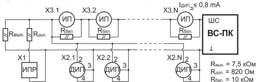
Рис 4. Схемы включения тепловых извещателей (типа ИП-105) в ШСП. Двухпороговый вариант работы пожарного ШС.
