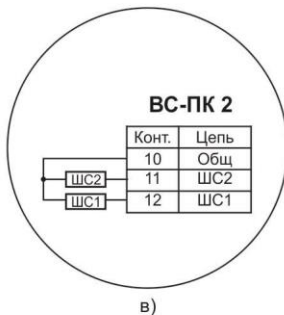
Рис.2. Схемы внешних соединений приборов: а) подключение прибора ВС-ПК8(Т)версия2.0; б) отличие подключения ВС-ПК4(Т)версия2.0; в) отличие подключения ВС-ПК2(Т)версия2.0.
