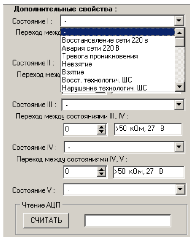
Рисунок 14. Задание состояний и порогов состояний для ШС типа 12
