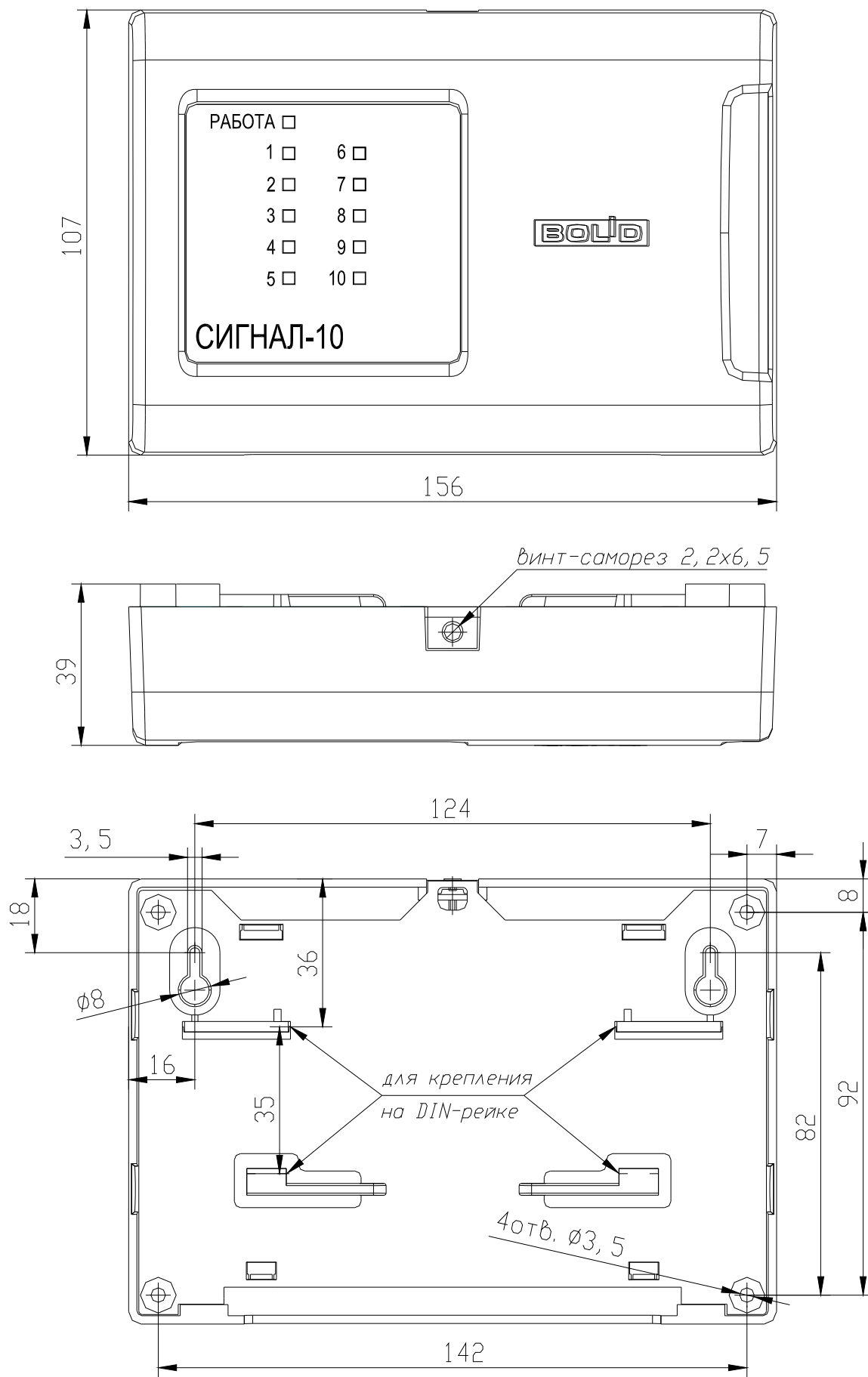
Рисунок 2. Габаритные и установочные размеры прибора Сигнал-10
