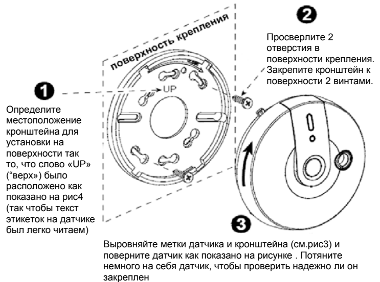
Рис 4. Монтаж
